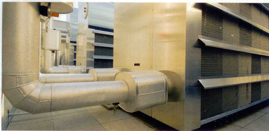
Blick in die Lüftungszentrale des Multiplex Kinos Pathé Küchlin in Basel, wo insgesamt drei luftgekühlte Kältemaschinen für ein angenehmes Klima in den acht Kinosälen sorgen. Foto IWB
